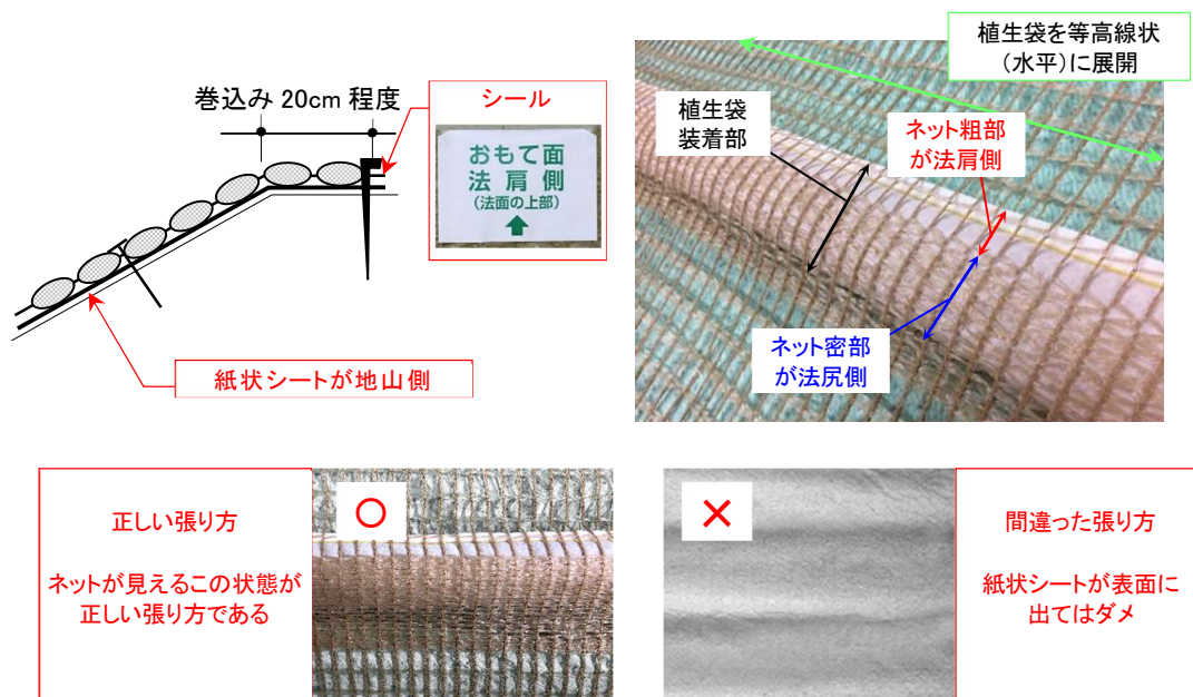
図1. マットの展開・施工方法
