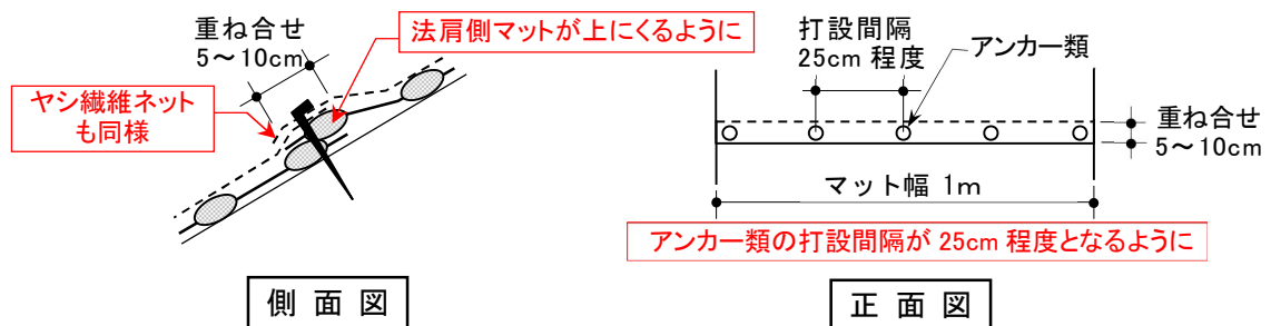
図 5. マット縦方向の重ね合わせとアンカー類の打設
