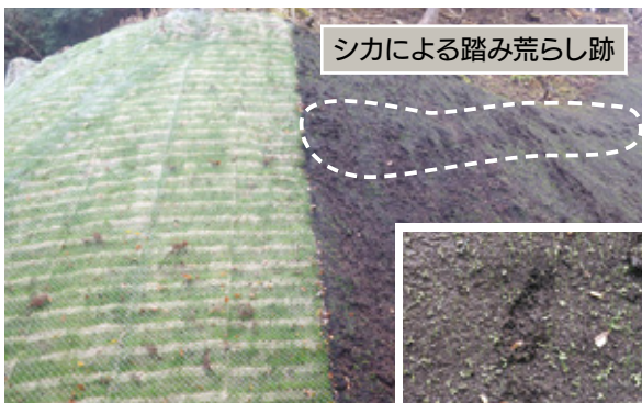
シカノン + ガンリョクマット 植生基材吹付工
