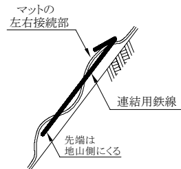
マツト左右接続部の連結方法(断面図)
