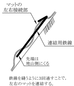
マット左右接続部の連結方法(断面図)
