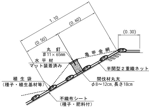
断面図 (1)
