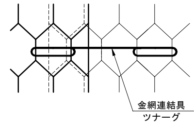
金網連結具詳細図
