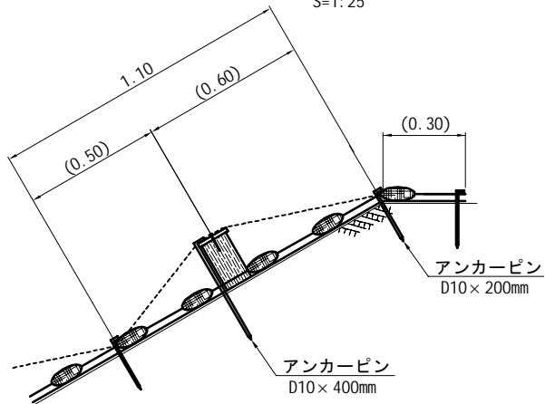
断面図 (2)
